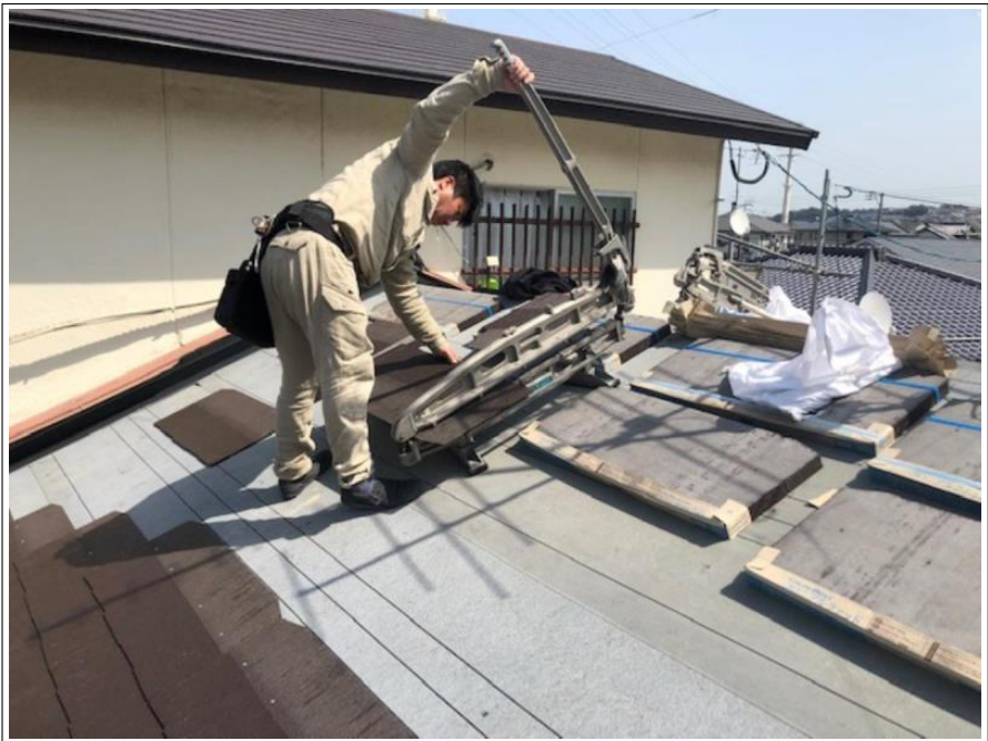
屋根 葺き替え工事
