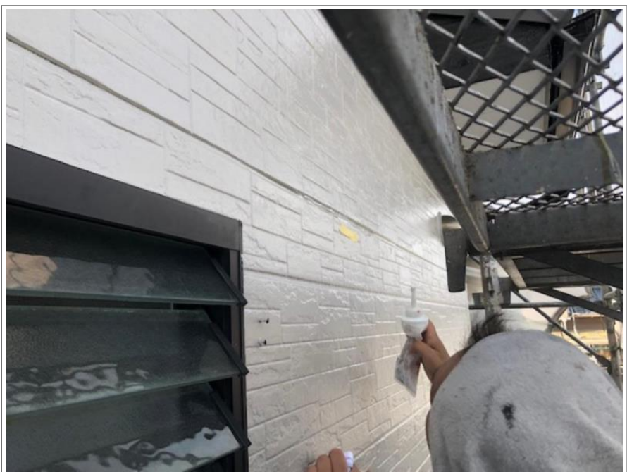
外壁 反り部コーキング
