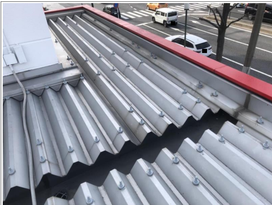
底屋根 ボルトキャップ取付け
