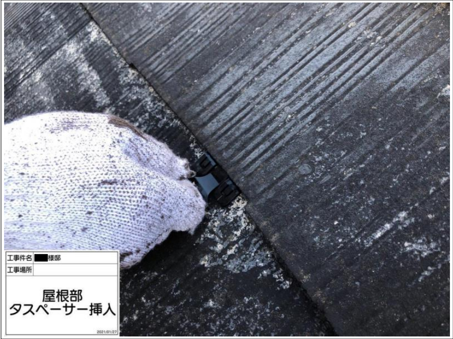
工事件名 ■棟部 工事場所 屋根部 タスペーサー挿入 2021/01/27
