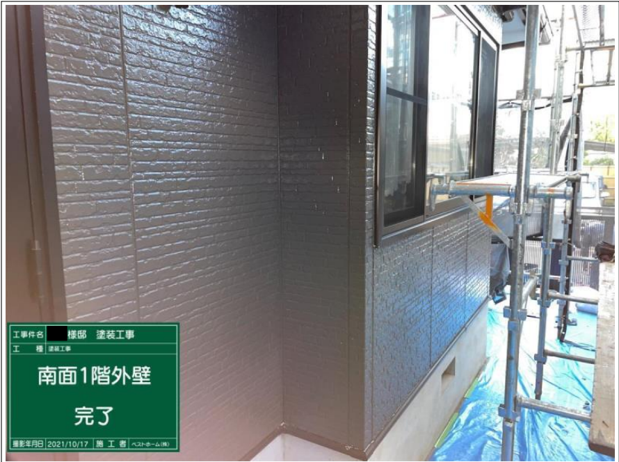
外壁 1階（南面）
