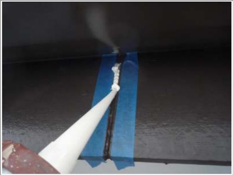
ハフ板コーキング補修施工中
