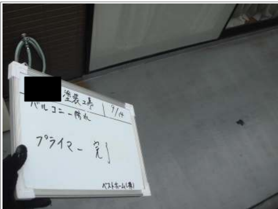
バルコニー防水 下塗り完了
