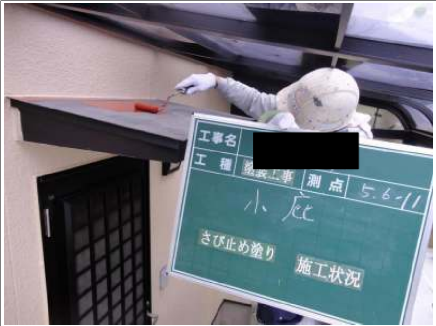
小底サビ止め施工状況
