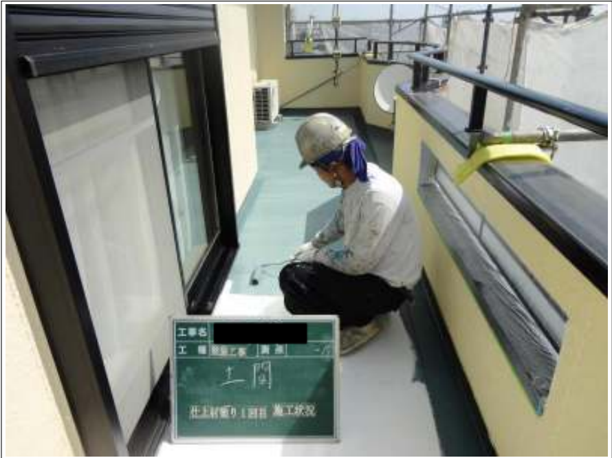
バルコニー上塗り施工状況（1回目）
