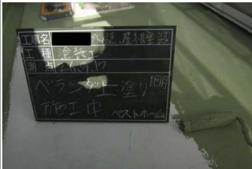
ベランダ塗装上塗り 1回目施工中
