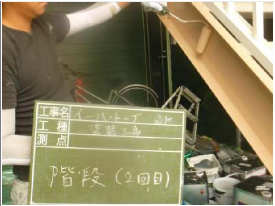
階段 上塗り施工中（2回目）
