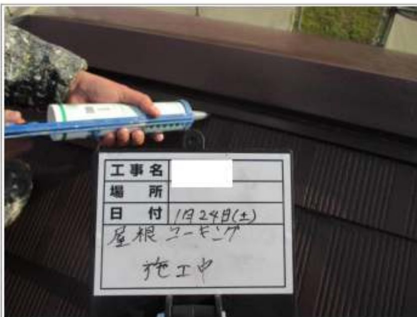
ラバー止め施工中
