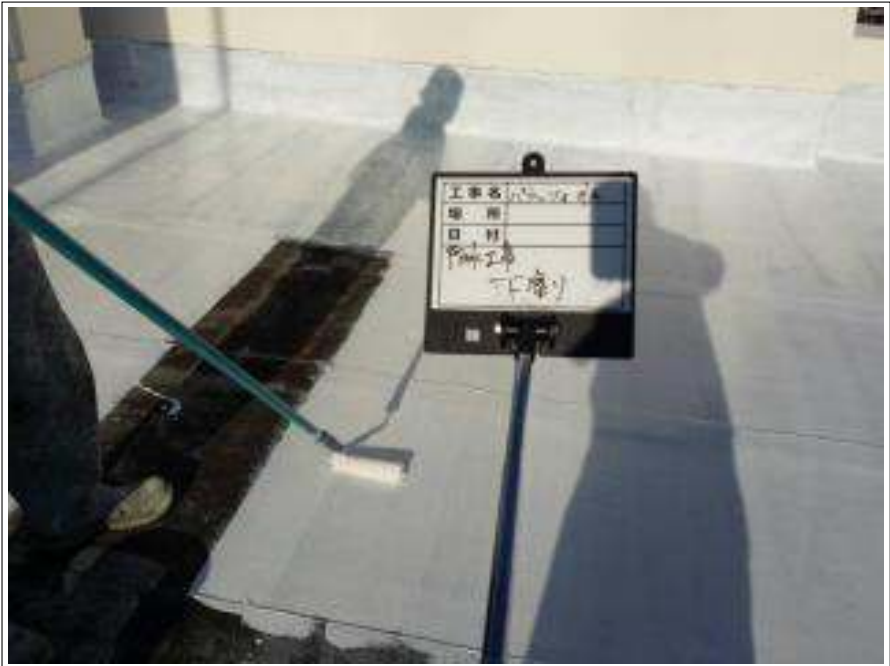
屋上防水部 下塗り施工中
