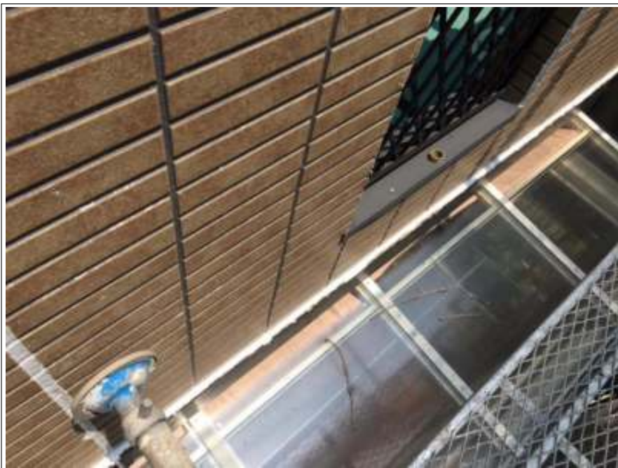
帯 シーリング補修 施工後
