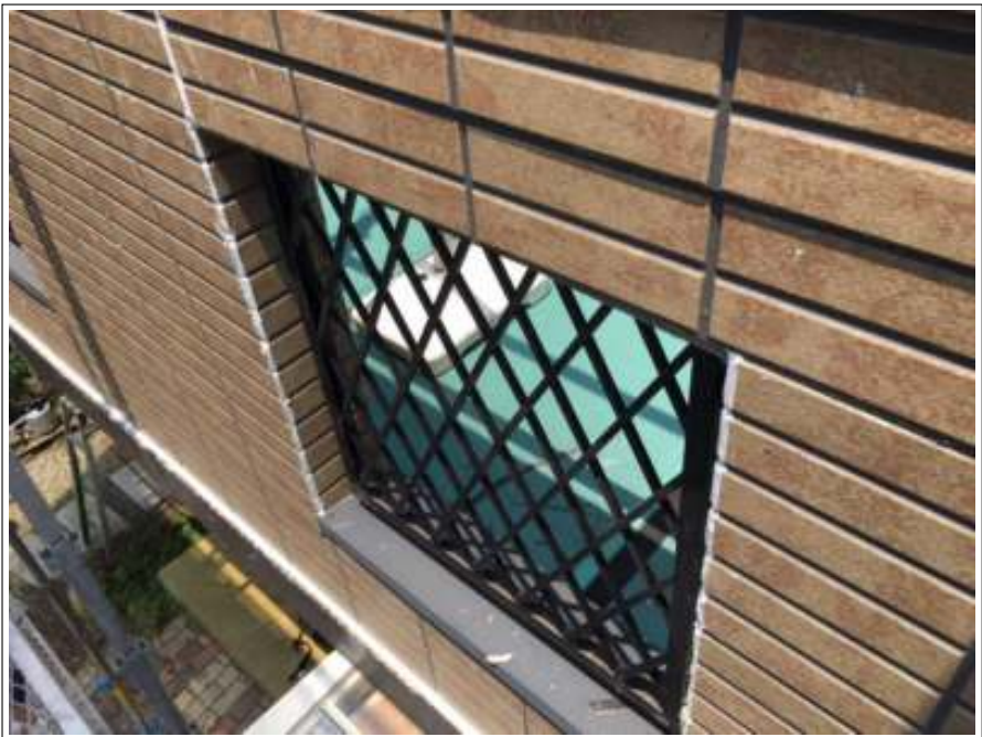
シーリング打ち増し 施工後
